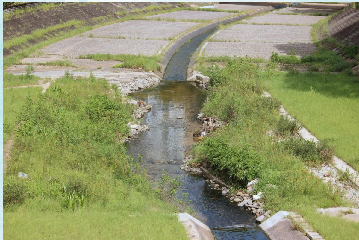
林村河下游生態改善試驗計劃河段
